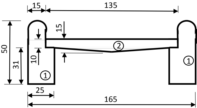
Vedere frontala
